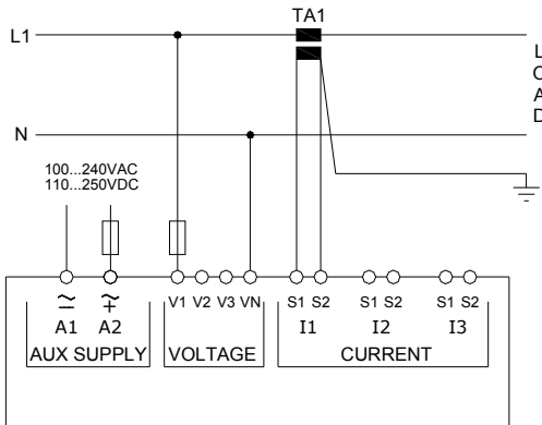
Podłączenie 1 fazowe Single phase connection P01.07 = L1-N
