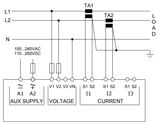
Podłączenie 2 fazowe 2 phase connection P01.07 = L1-N-L2
